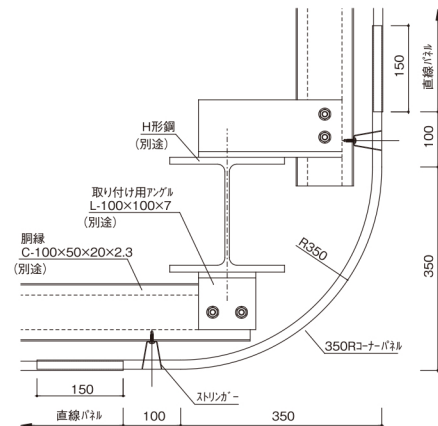
350R コーナーパネル納まり図
