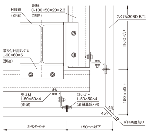
30BD-E パネル横貼りコーナー納まり図
