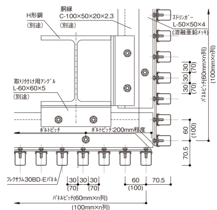
30BD-E パネル縦貼りコーナー納まり図
