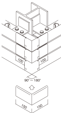
V,SS タイプコーナーパネル
