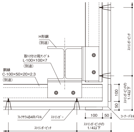
コーナーパネル納まり図
