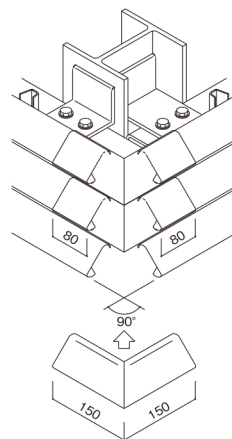
SL,EL タイプコーナーパネル
