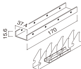
ストリングースプライス(EL用)
