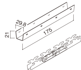
ストリンガースプライス(V、R、H、SL用)
