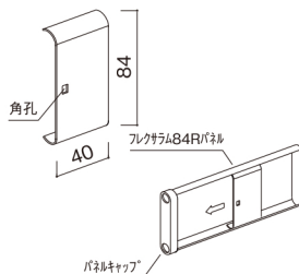
パネルキャップホルダー
