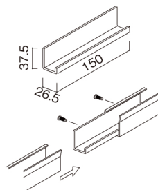
ボーダースプライス(ボーダー26用)
