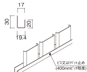
ボーダー 17 (V、R、SS用)
