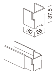
ボーダーエンドキャップ(ボーダー 26 用)
