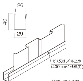
ボーダー 26 (R用)
