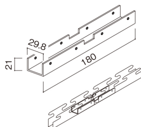
ストリングースプライス(SS用)
