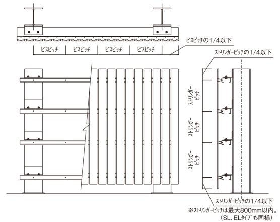
ストリンガー V,SS タイプ パネル縦貼り姿図
