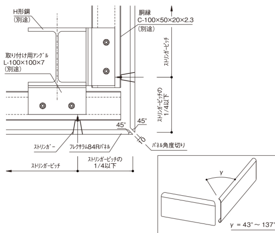
パネル角度切り納まり図(ストリンガー V,SS タイプ)
