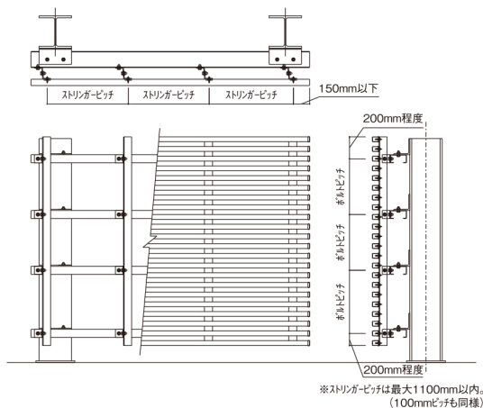
30BD-E パネル(60mmピッチ)横貼り姿図
