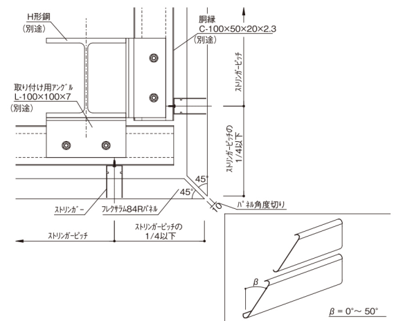
パネル角度切り納まり図(ストリンガー H,SL,EL タイプ)
