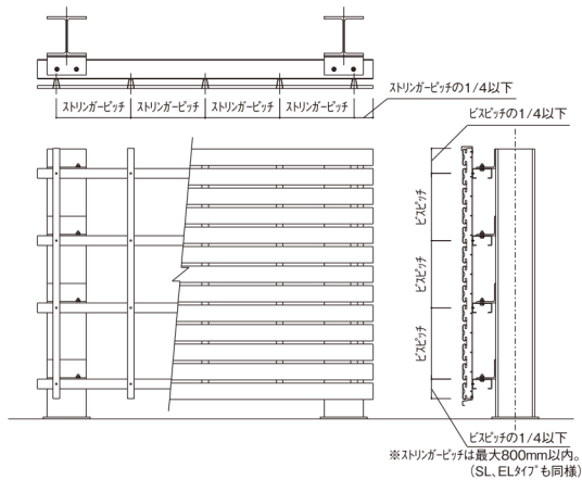
ストリンガー V,SS タイプ パネル横貼り姿図
