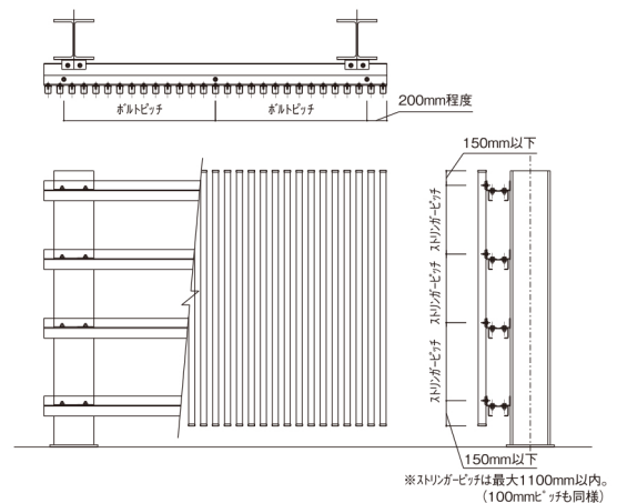
30BD-E パネル(60mmピッチ)縦貼り姿図
